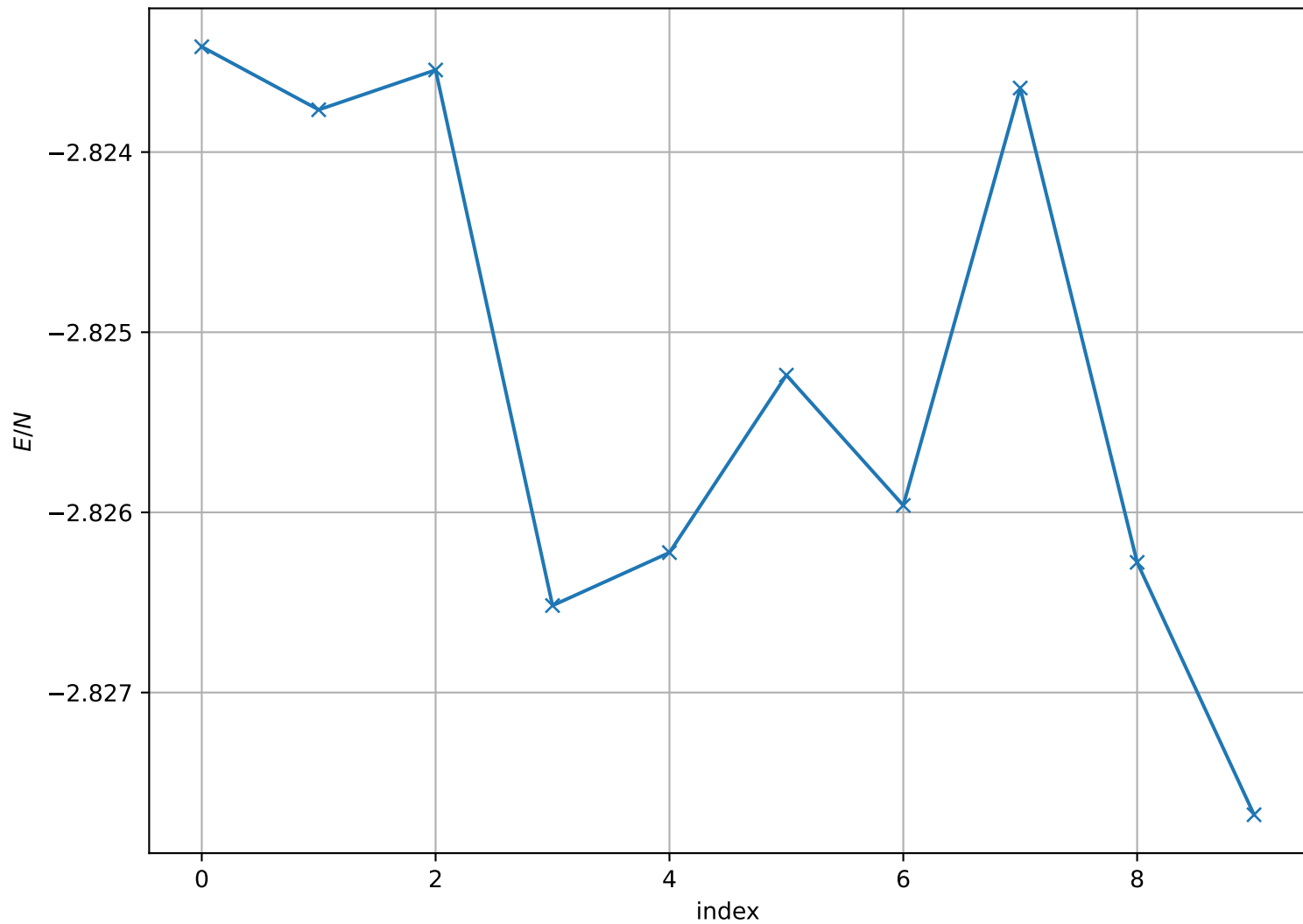
Energy per Site at T = 1.000e - 01 , L = 32
