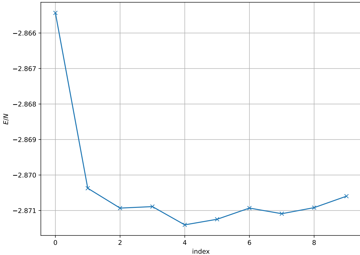
Energy per Site at T = 1.000e - 02 , L = 32
