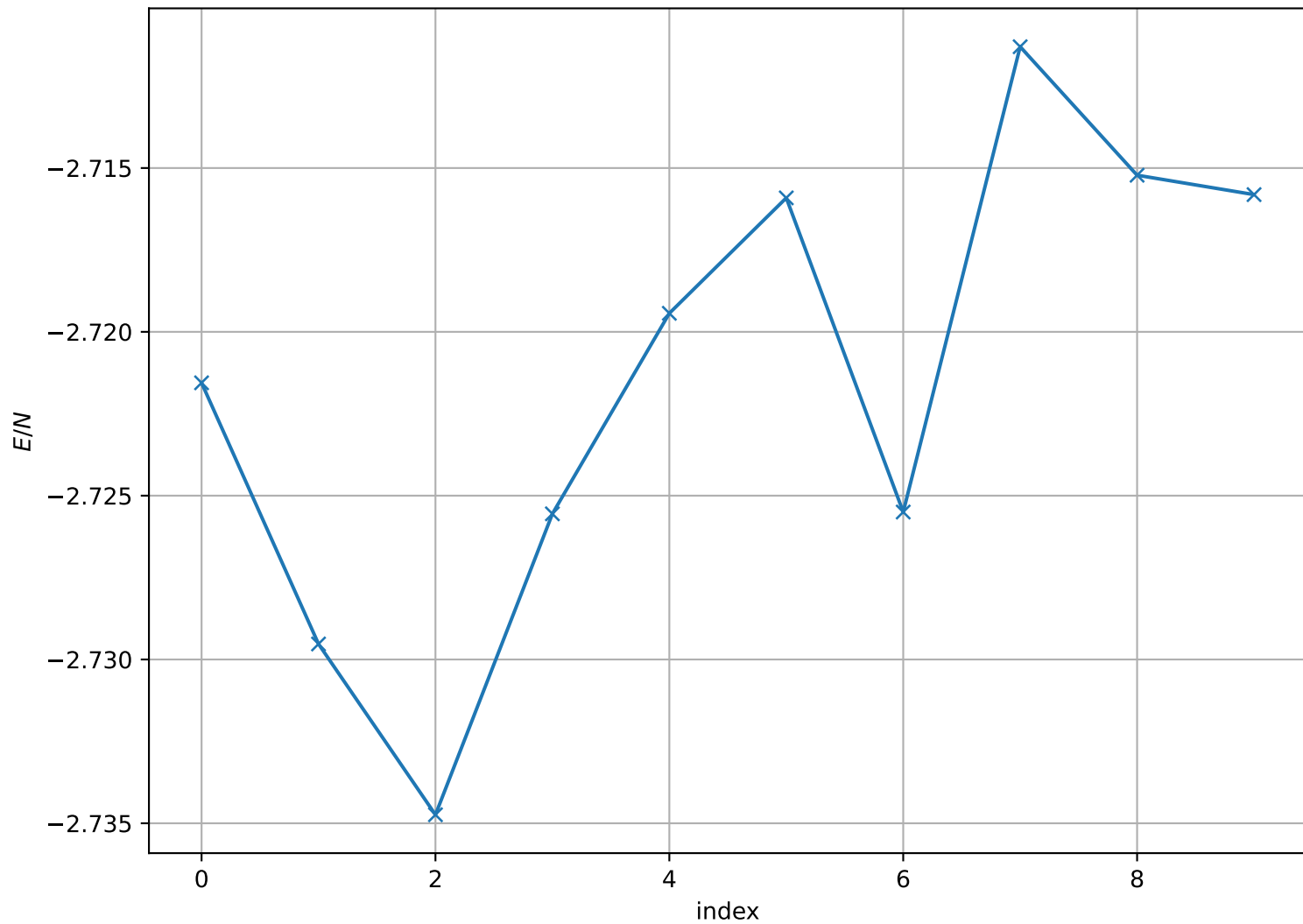
Energy per Site at T = 3.000e - 01 , L = 32
