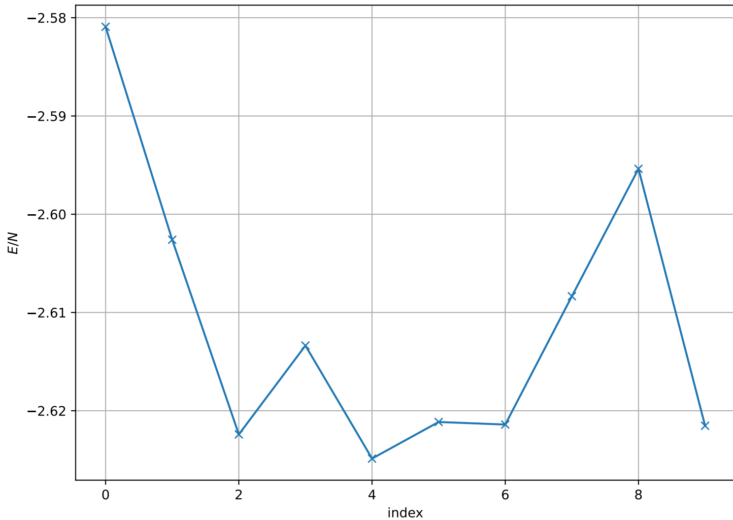
Energy per Site at T = 5.000e - 01 , L = 32
