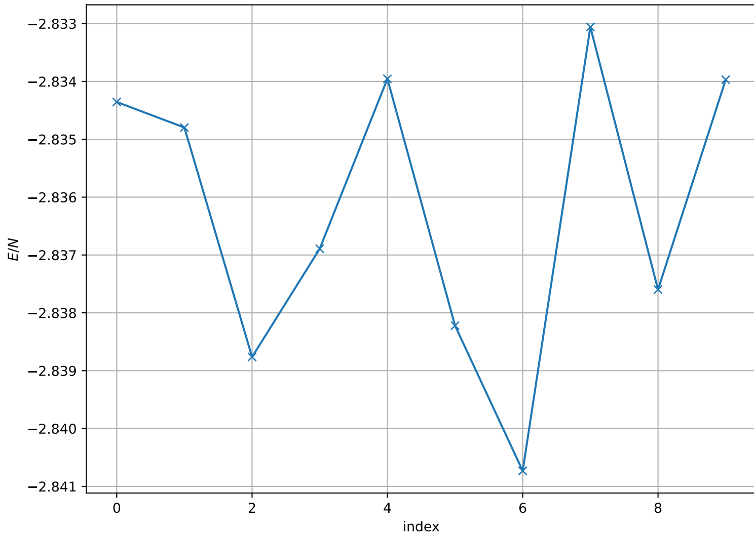
Energy per Site at T = 2.000e - 01 , L = 64
