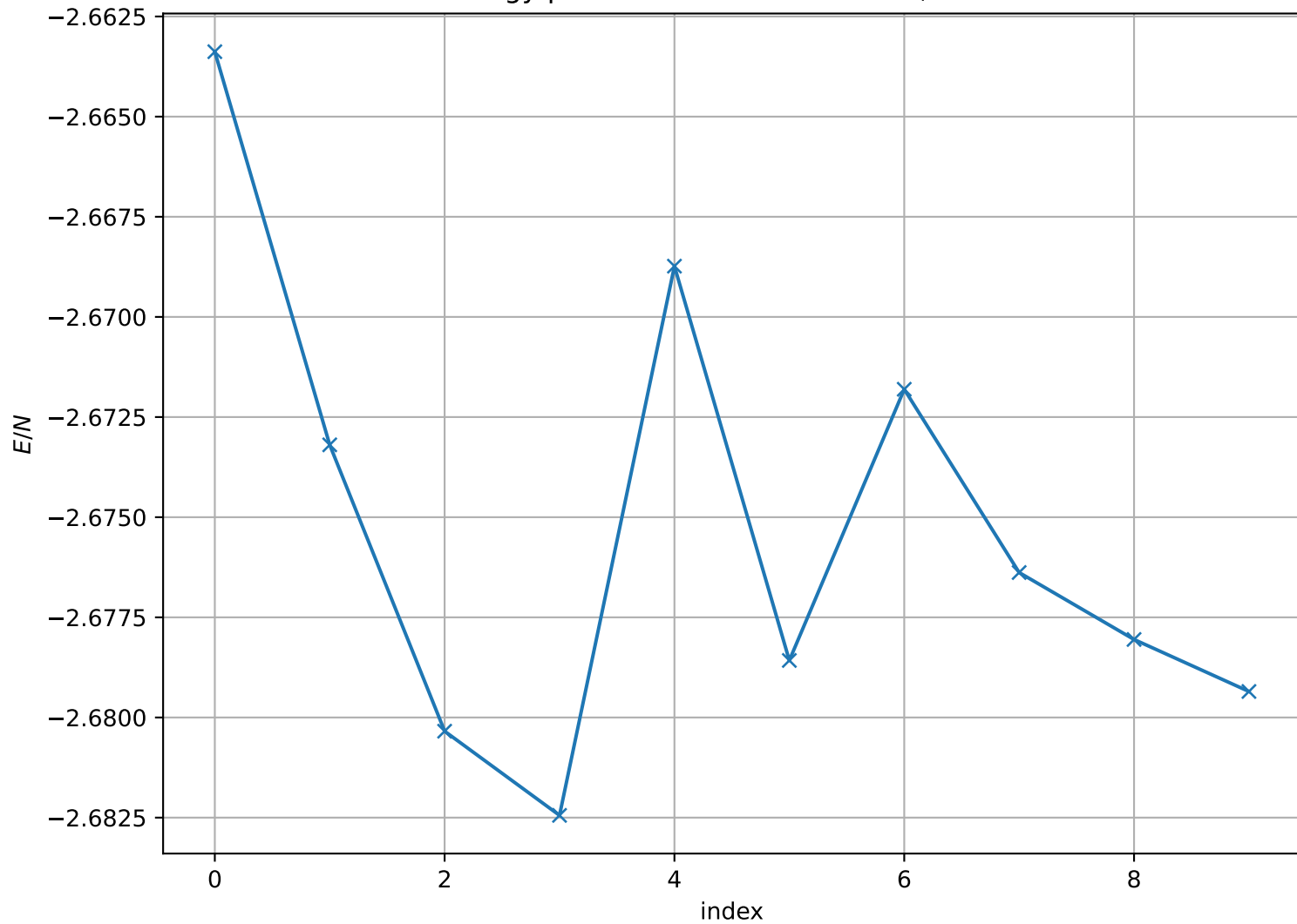
Energy per Site at T = 5.000e - 01 , L = 64
