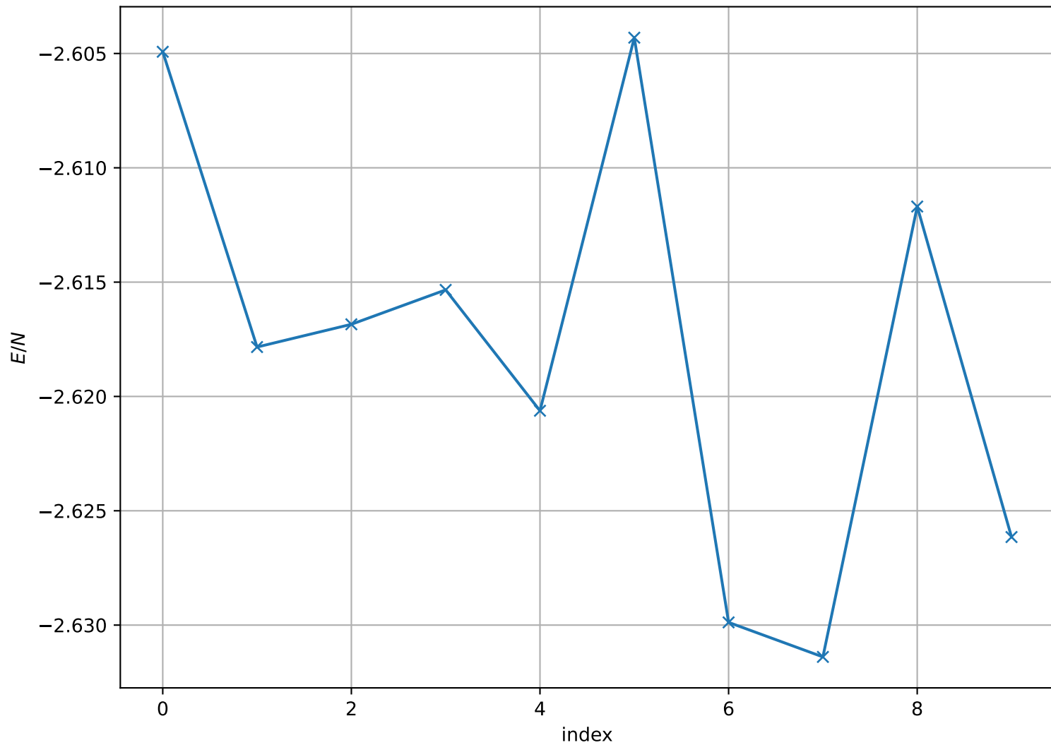
Energy per Site at T = 6.000e - 01 , L = 64
