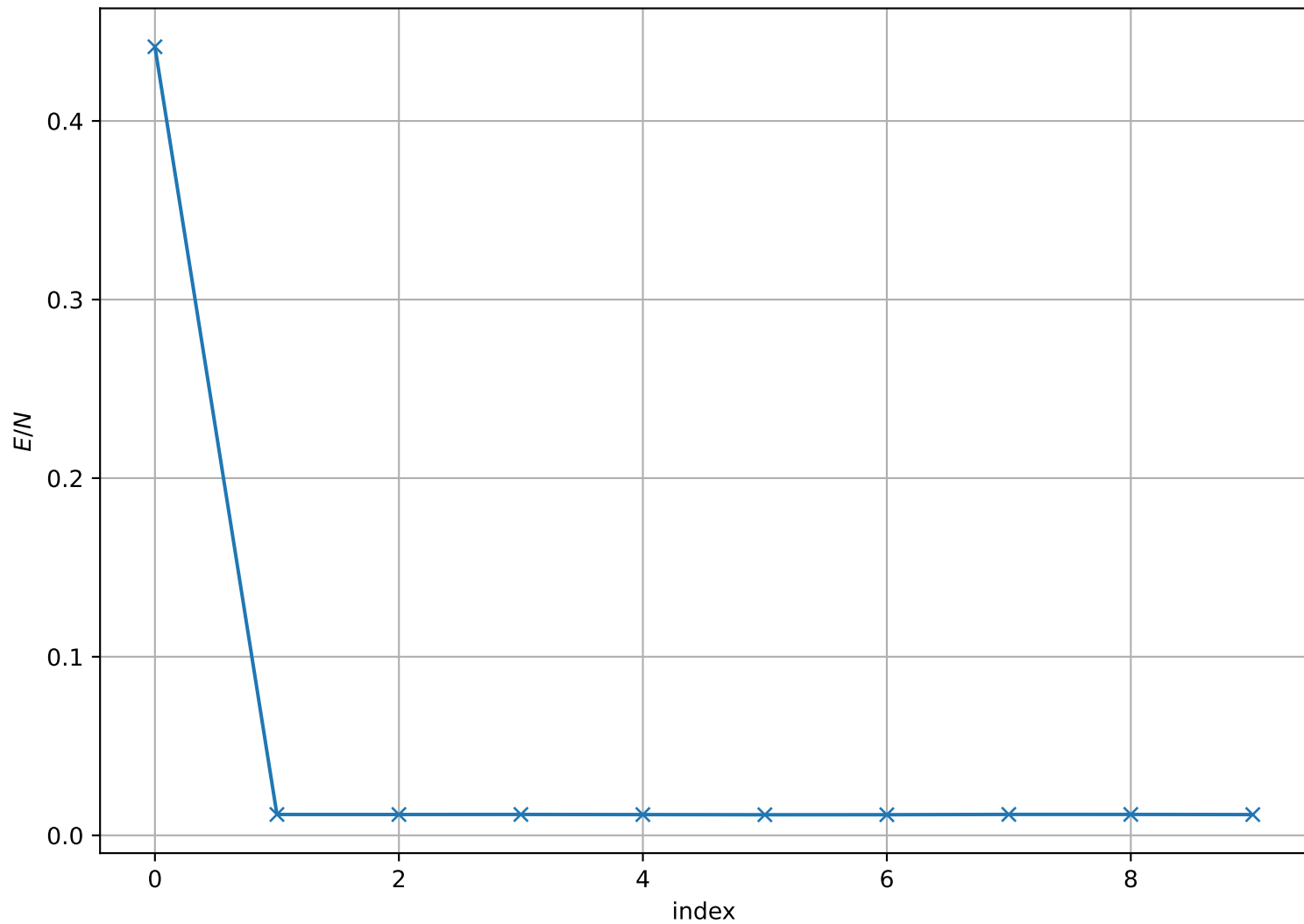
Energy per Site at T = 1.000e - 02 , L = 128
