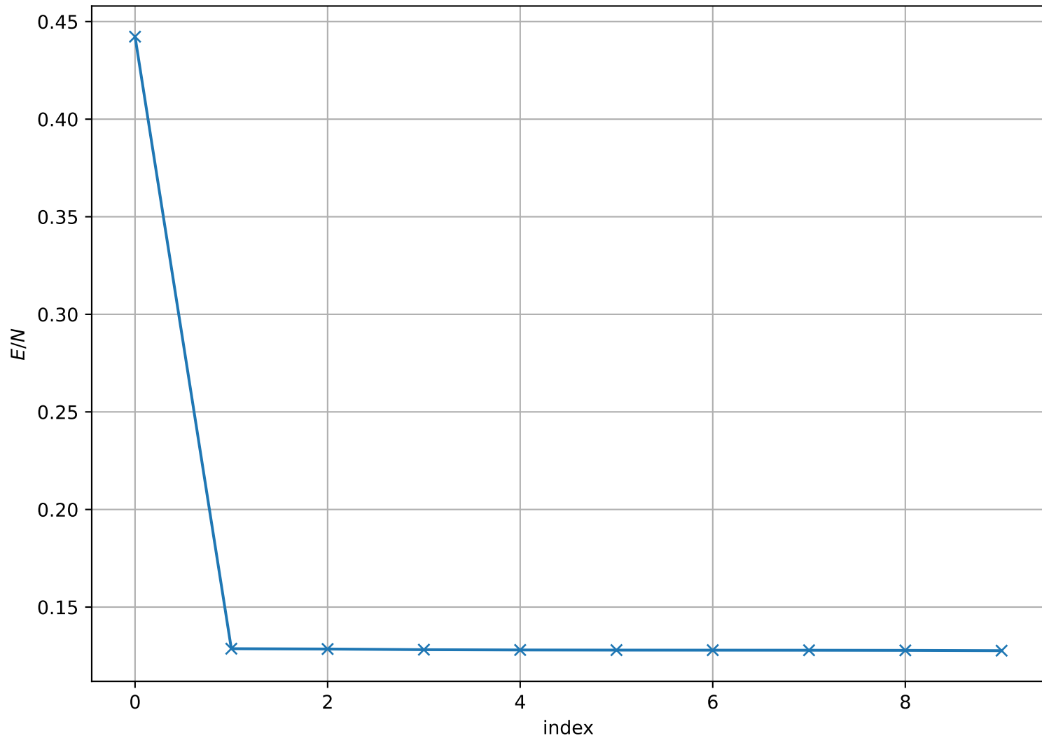
Energy per Site at T = 1.000e - 05 , L = 128
