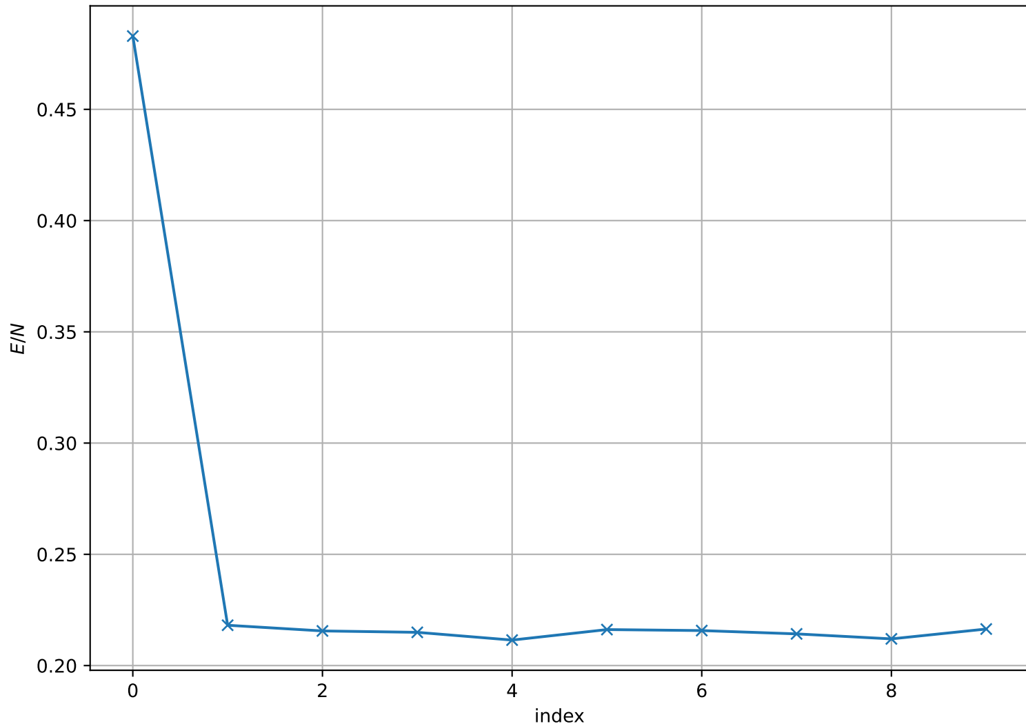
Energy per Site at T = 1.500e - 01 , L = 128
