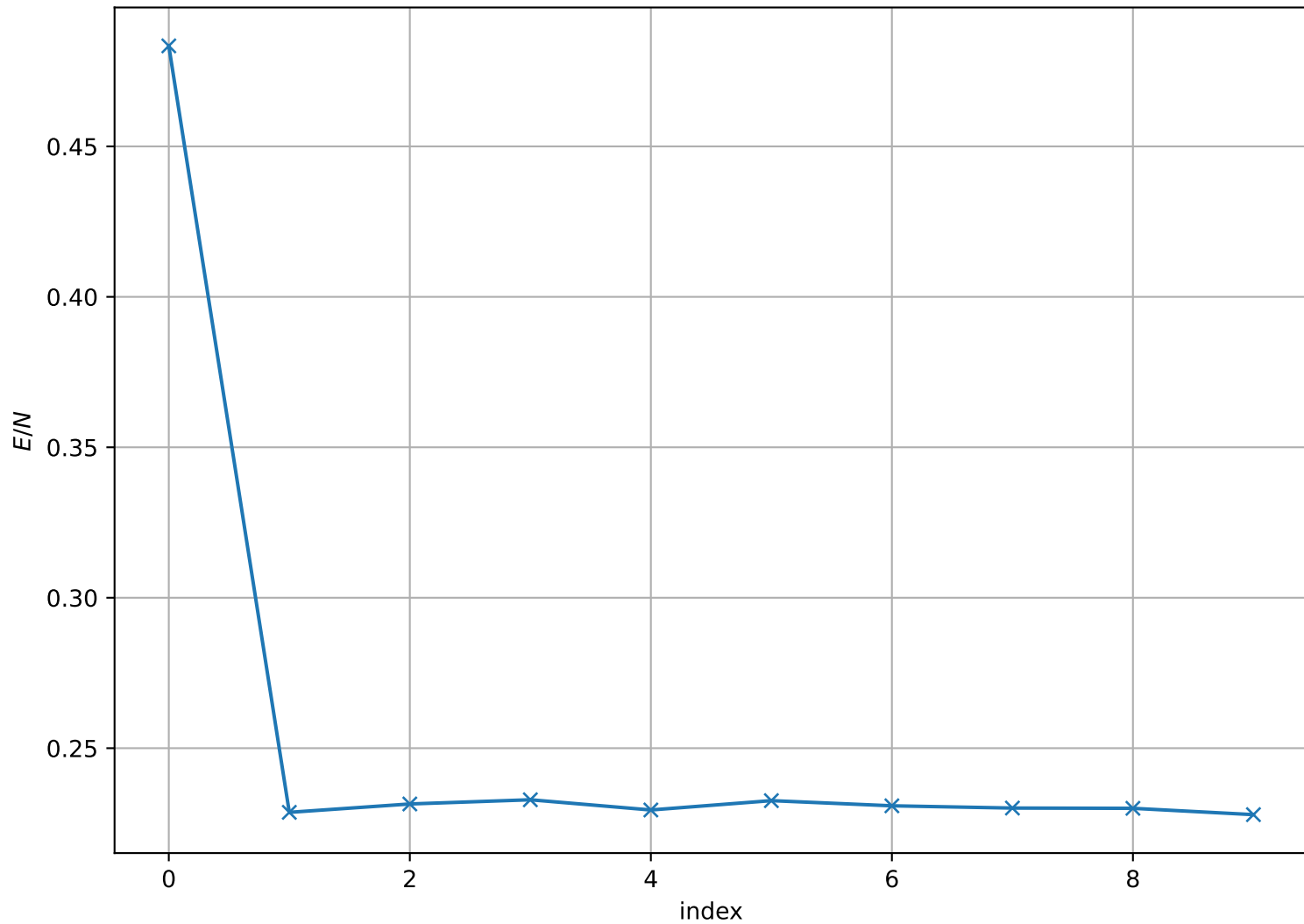
Energy per Site at T = 1.600e - 01 , L = 128
