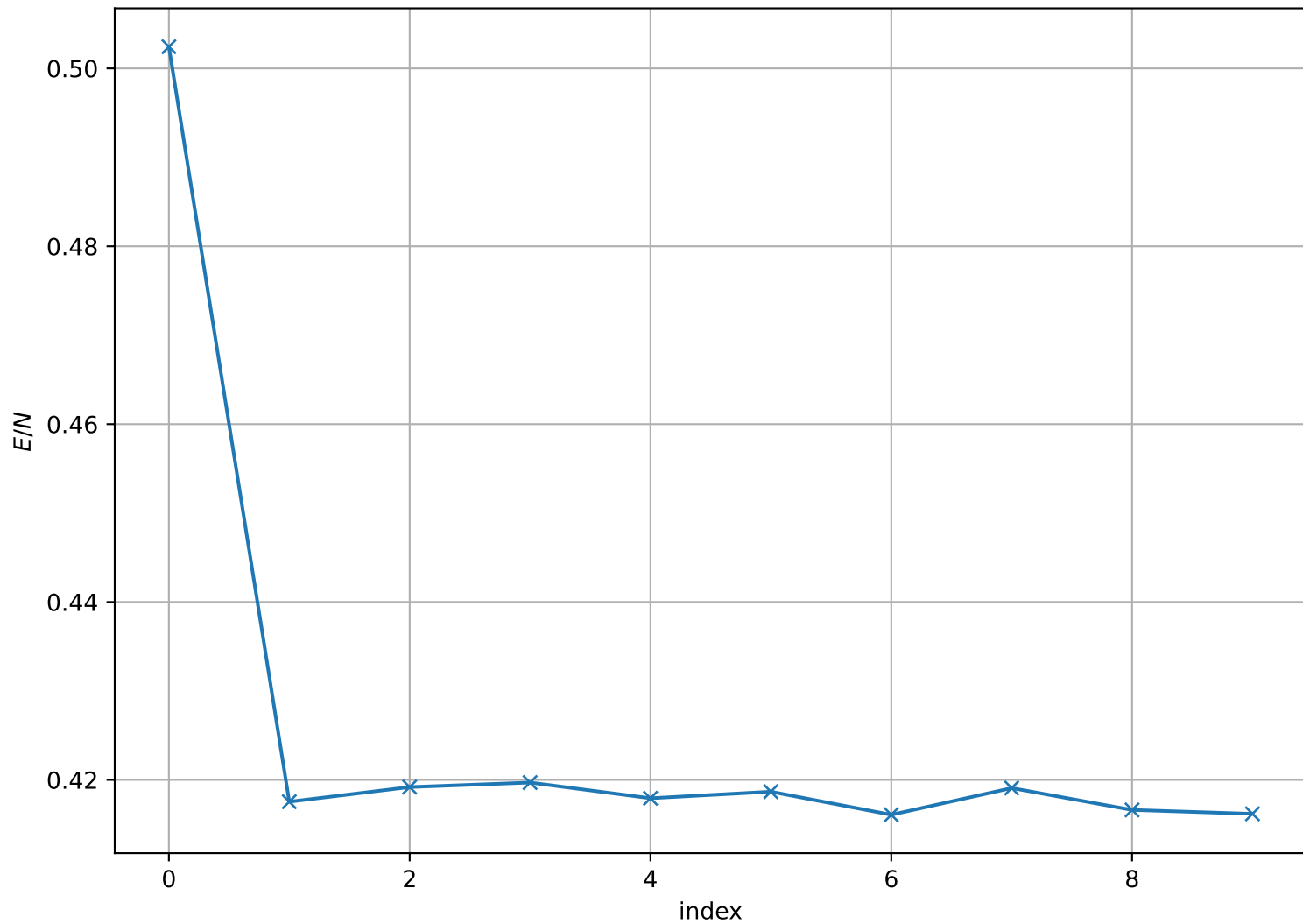
Energy per Site at T = 2.500e - 01 , L = 128
