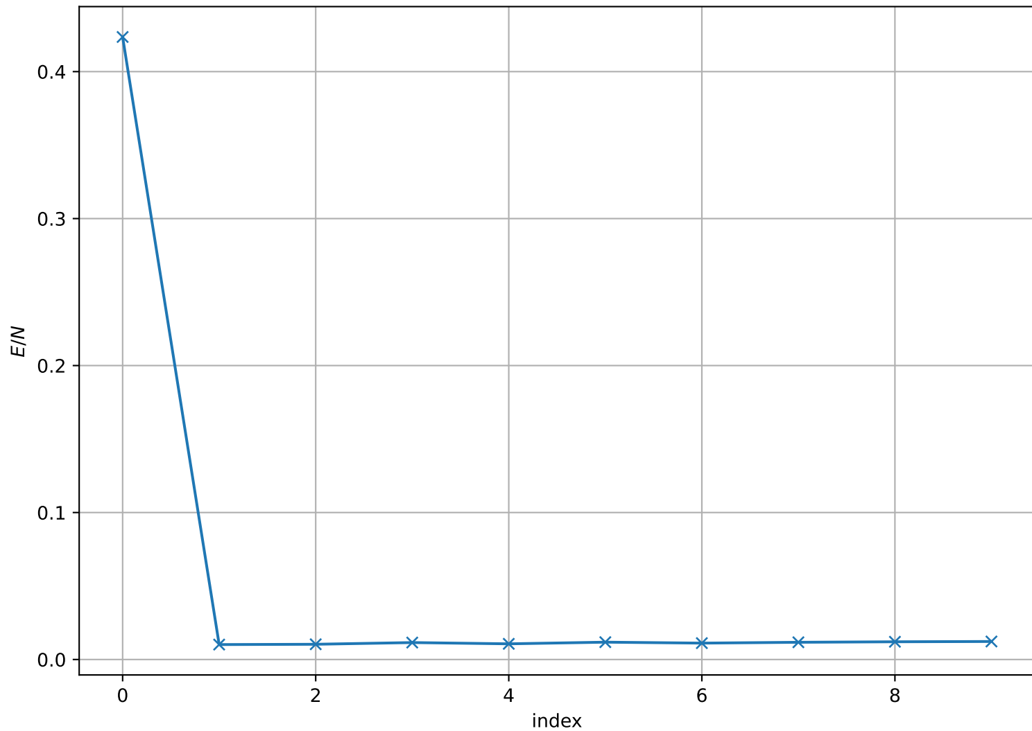
Energy per Site at T = 1.000\text{e} - 02 , L = 16
