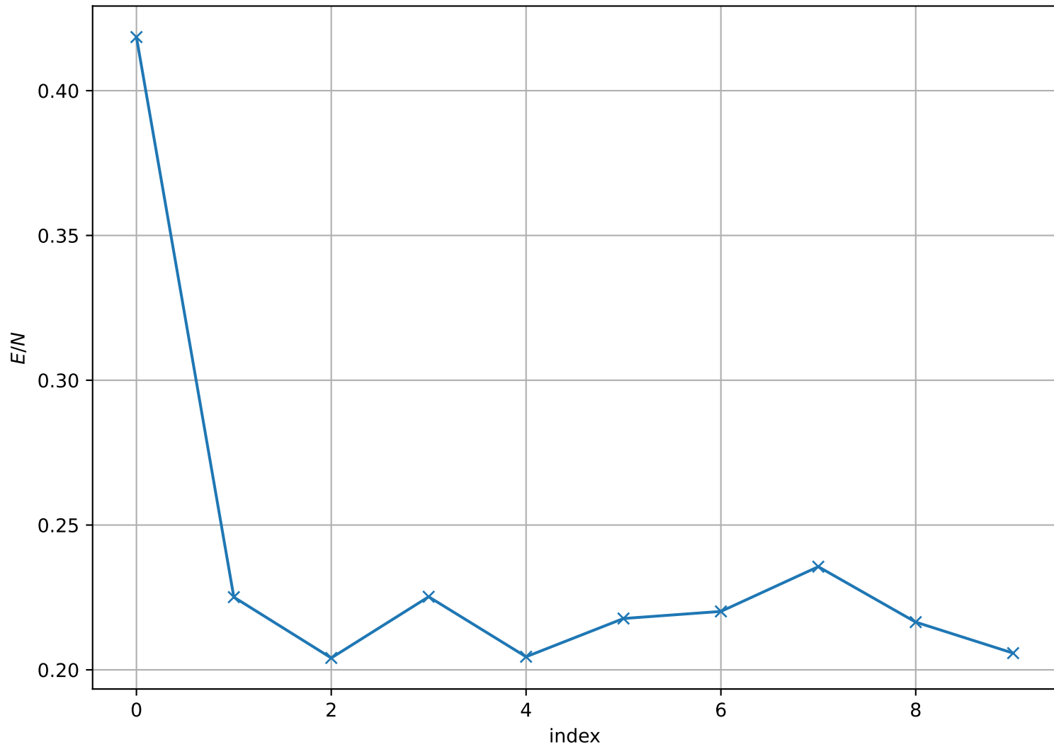
Energy per Site at T = 1.500e - 01 , L = 16
