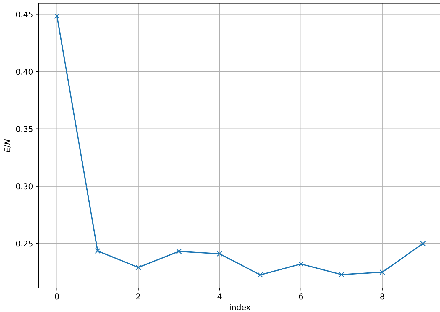
Energy per Site at T = 1.600e - 01 , L = 16
