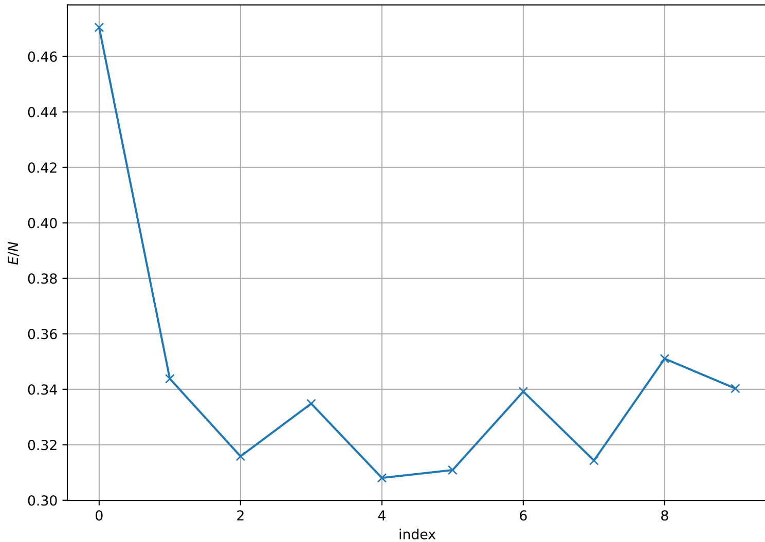
Energy per Site at T = 2.050e - 01 , L = 16
