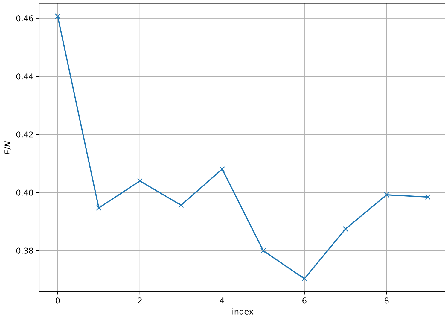
Energy per Site at T = 2.500e - 01 , L = 16
