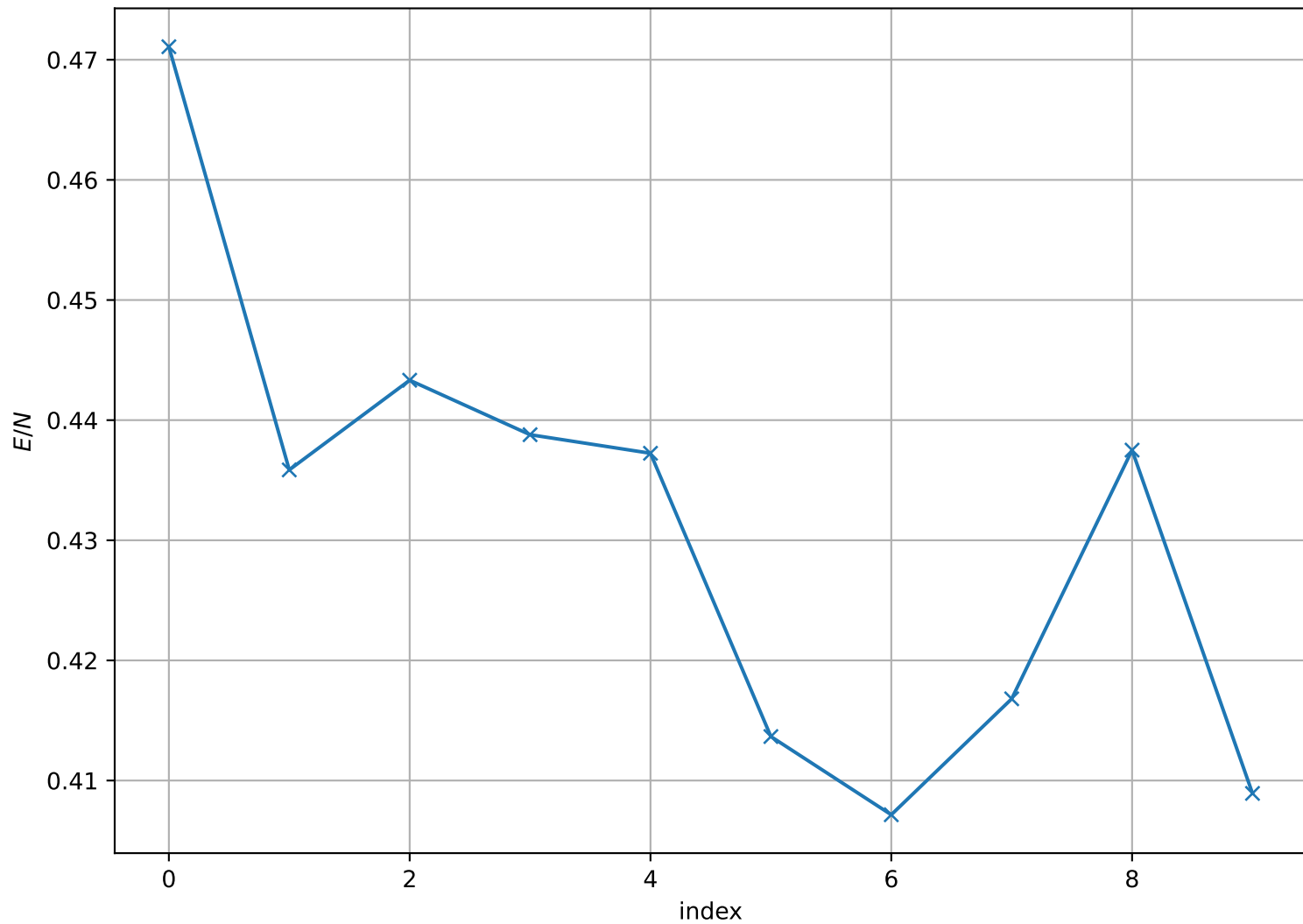
Energy per Site at T = 3.000e - 01 , L = 16
