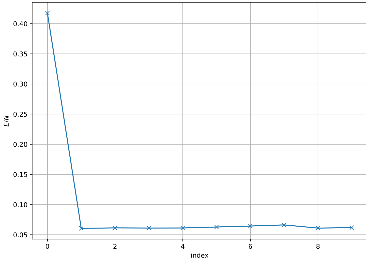
Energy per Site at T = 5.000e - 02 , L = 16
