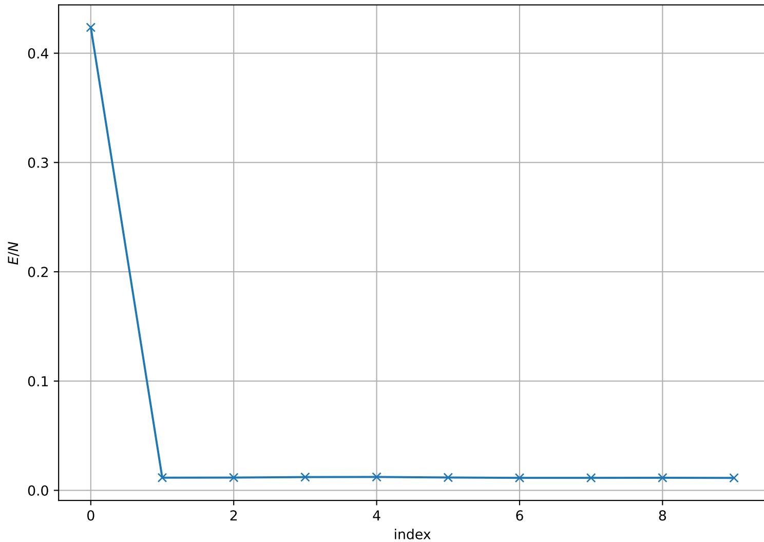
Energy per Site at T = 1.000\text{e} - 02 , L = 32
