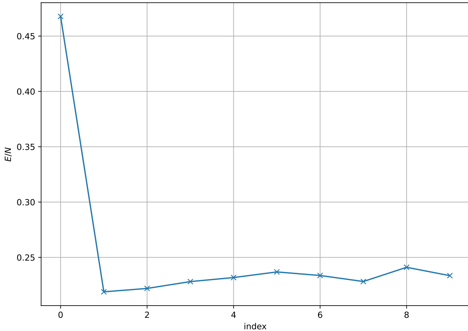
Energy per Site at T = 1.600e - 01 , L = 32
