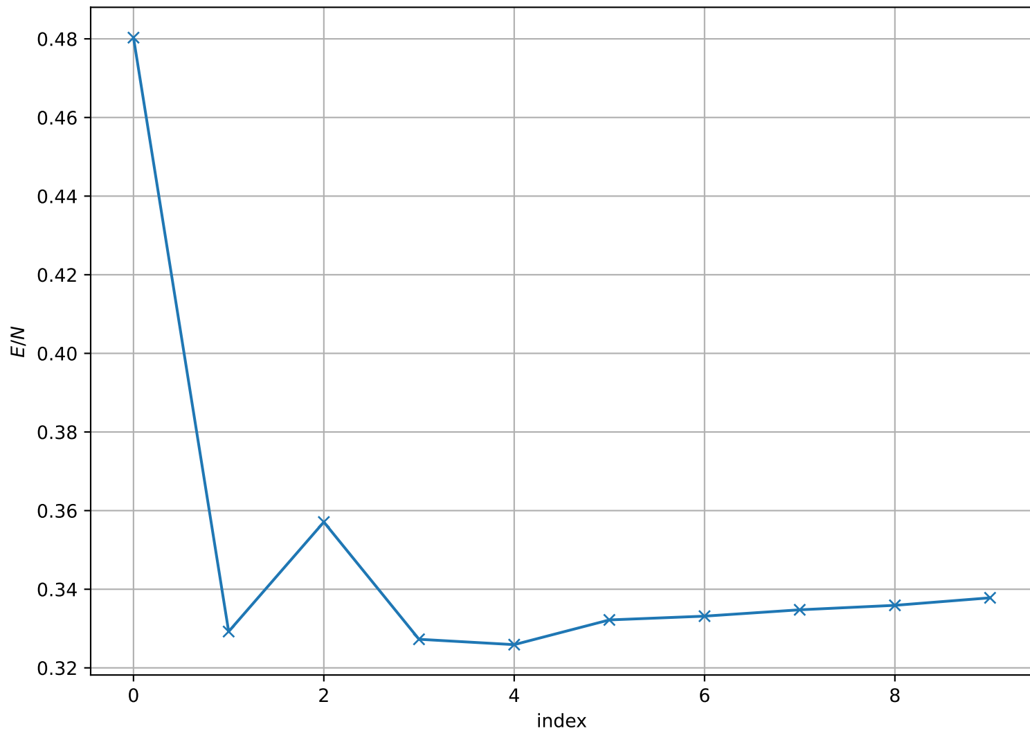
Energy per Site at T = 2.050e - 01 , L = 32
