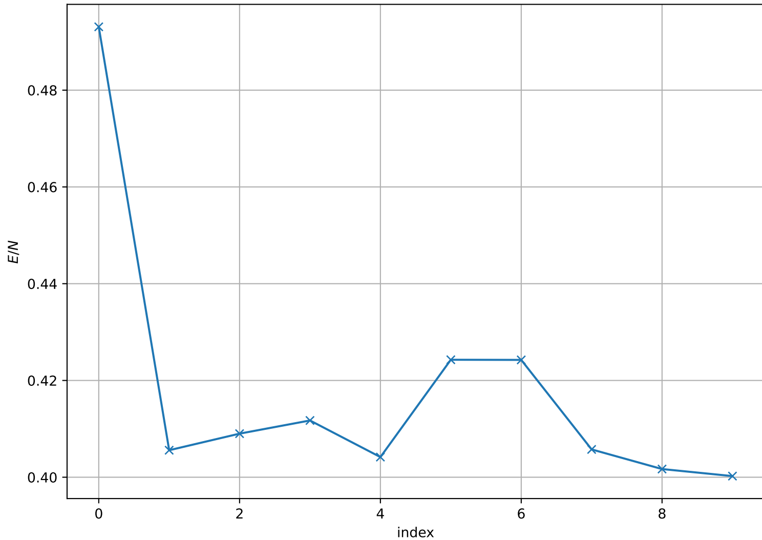
Energy per Site at T = 2.500e - 01 , L = 32
