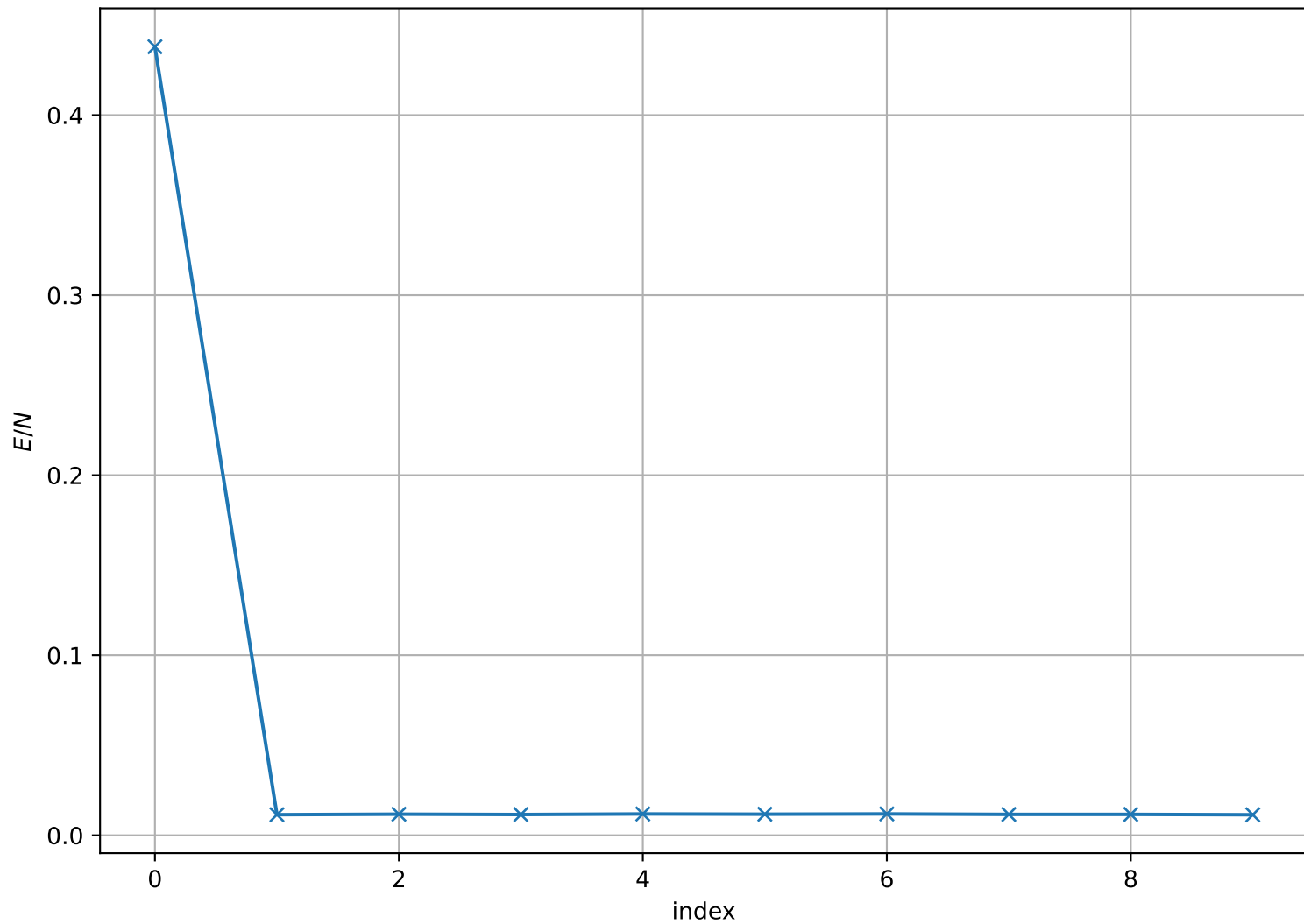
Energy per Site at T = 1.000\text{e} - 02 , L = 64
