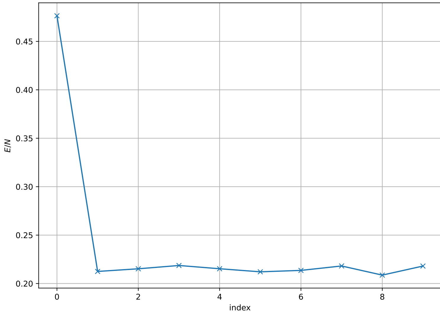
Energy per Site at T = 1.500e - 01 , L = 64
