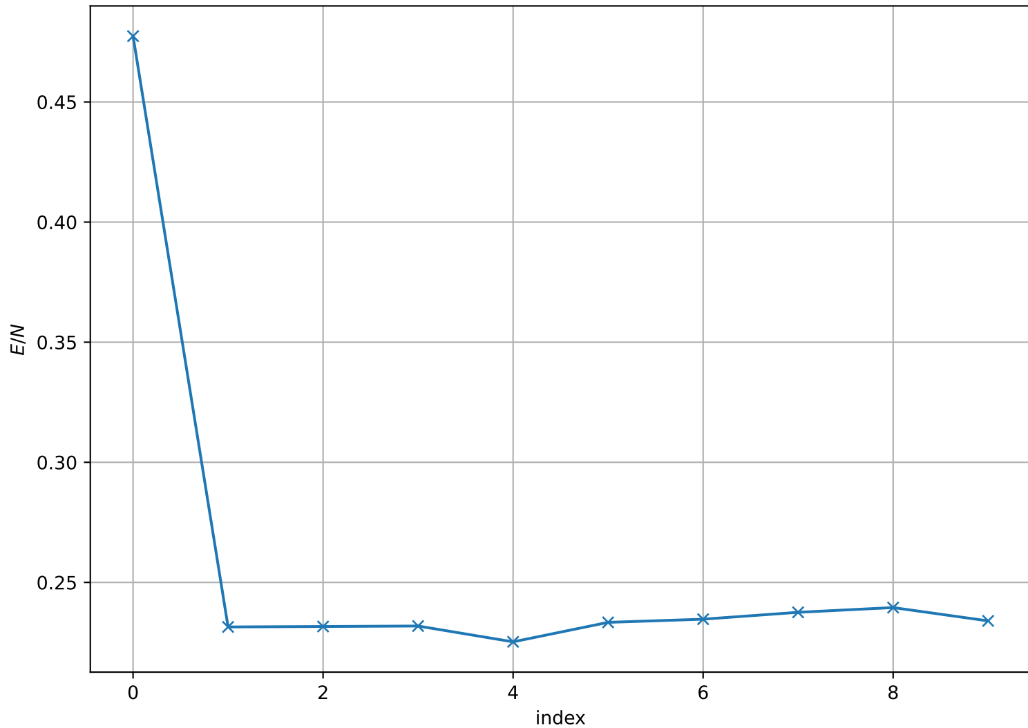
Energy per Site at T = 1.600e - 01 , L = 64
