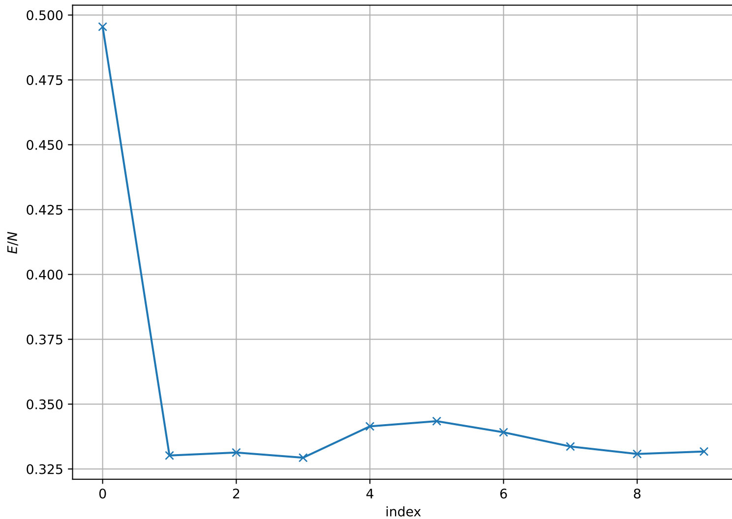
Energy per Site at T = 2.050e - 01 , L = 64
