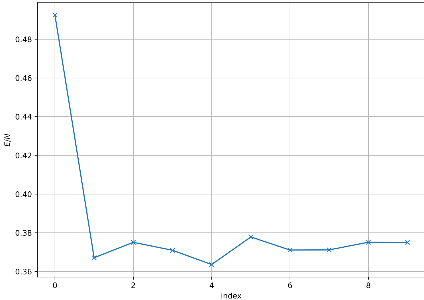
Energy per Site at T = 2.200e - 01 , L = 64
