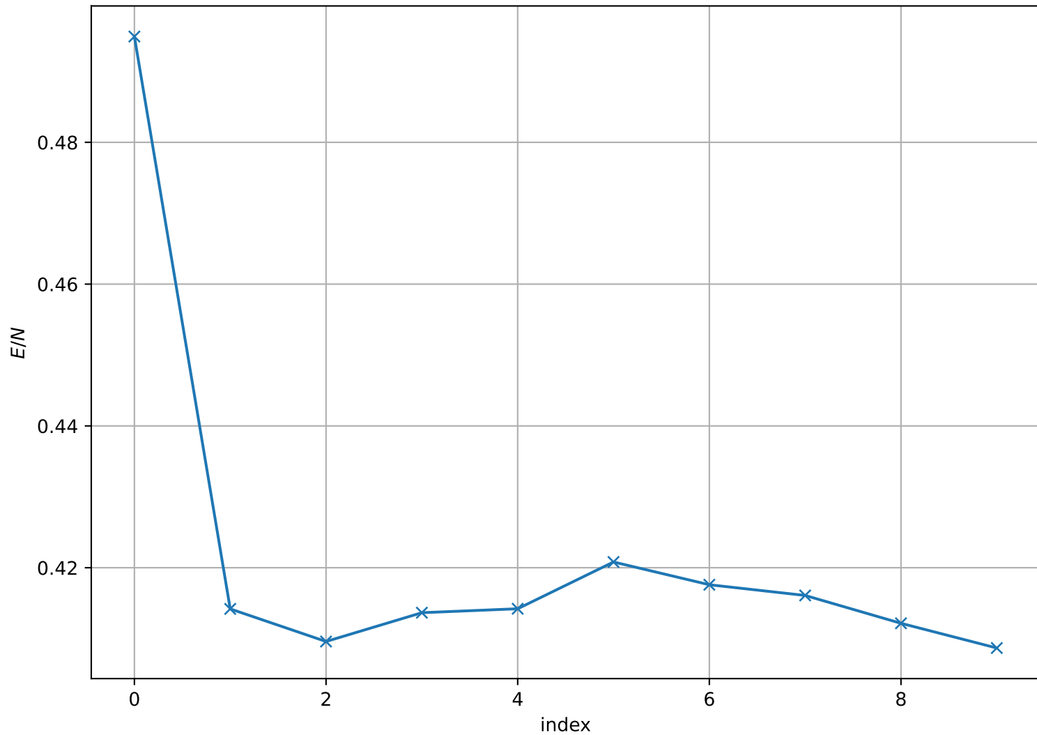
Energy per Site at T = 2.500e - 01 , L = 64
