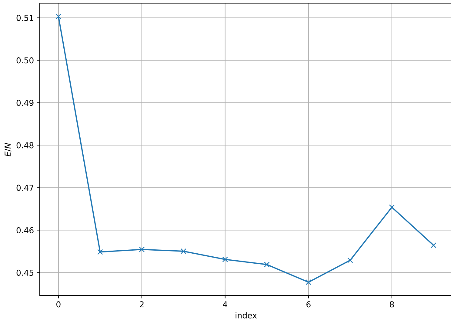
Energy per Site at T = 3.000e - 01 , L = 64
