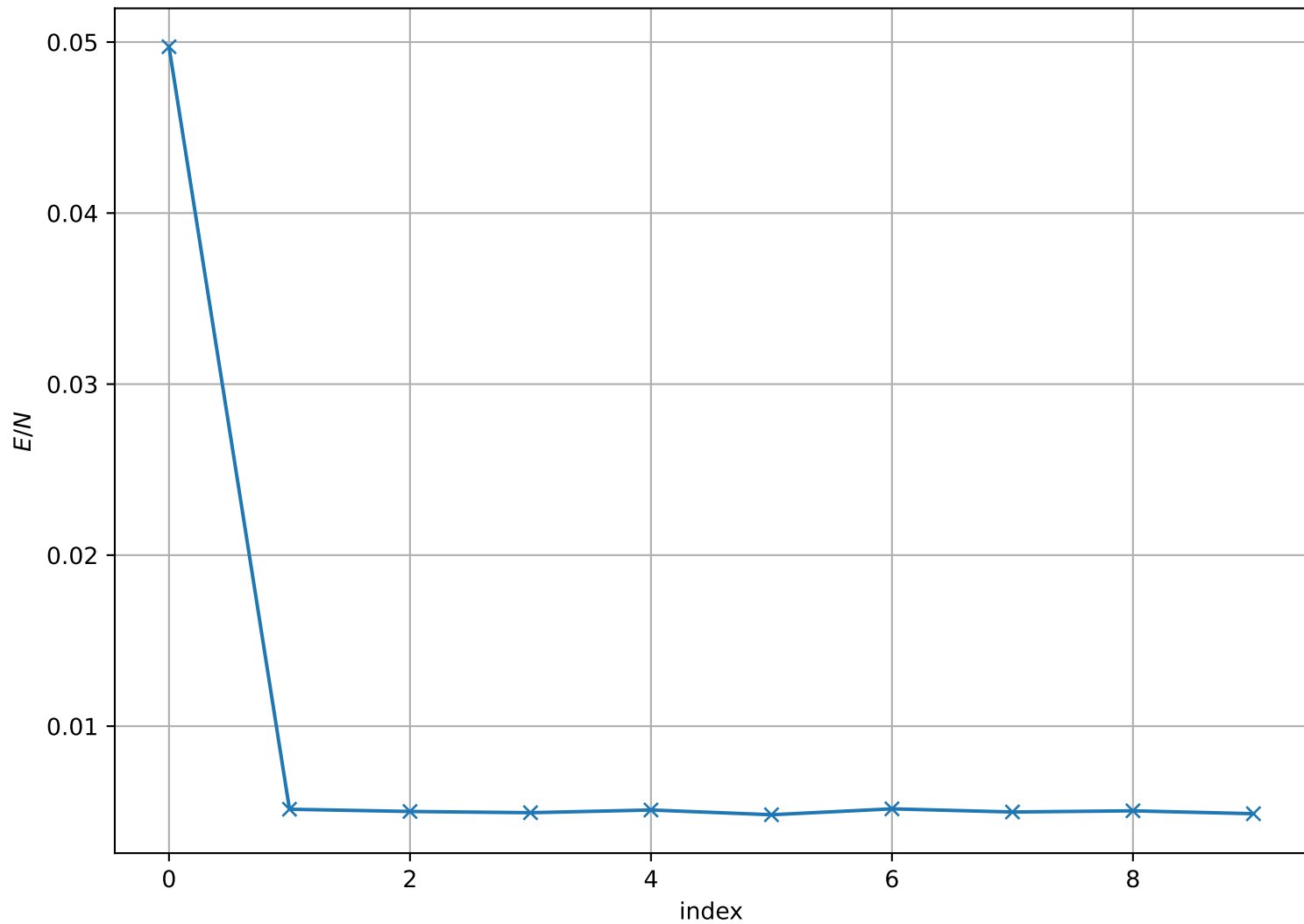
Energy per Site at T = 1.000e - 02 , L = 64
