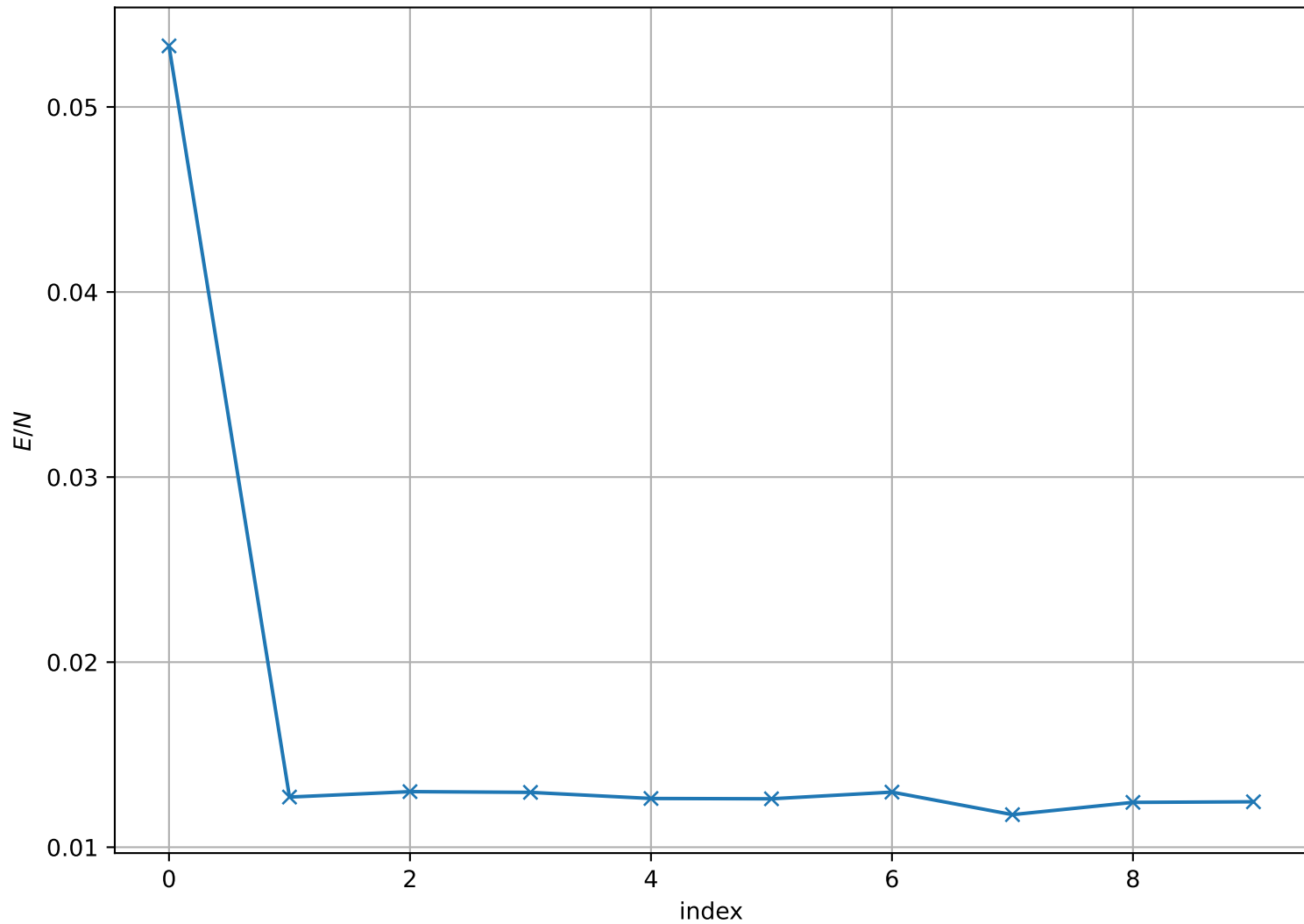
Energy per Site at T = 2.500e - 02 , L = 64
