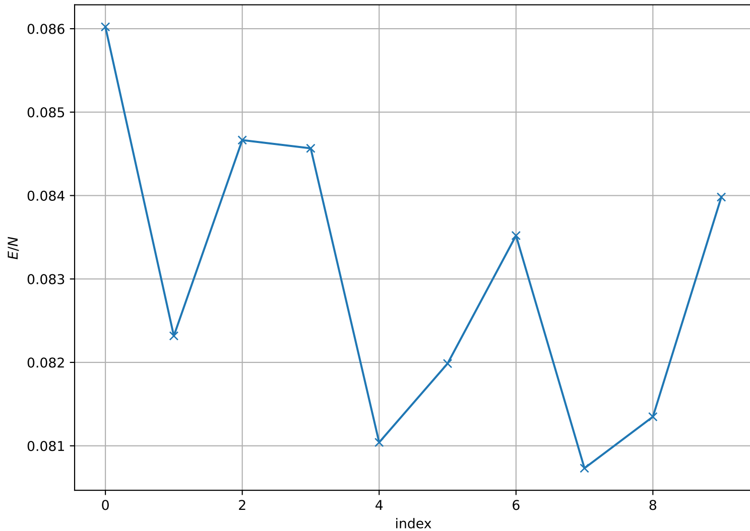
Energy per Site at T = 8.000e - 01 , L = 64
