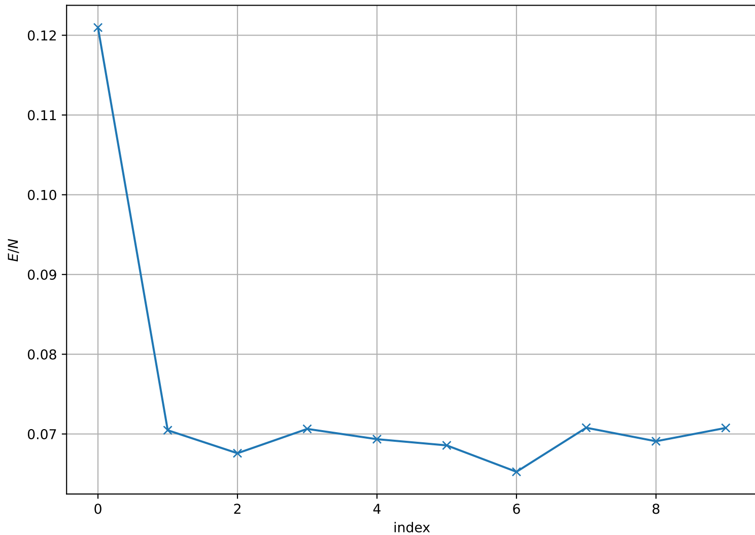
Energy per Site at T = 1.500e - 01 , L = 32
