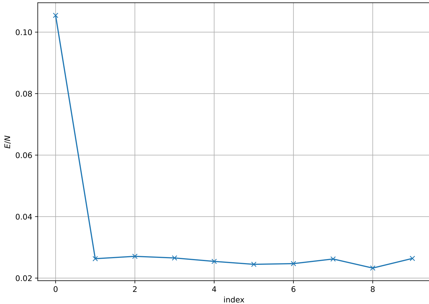
Energy per Site at T = 5.000e - 02 , L = 32
