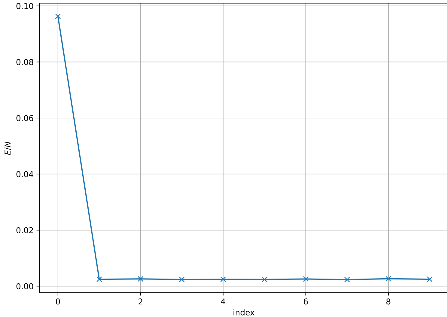
Energy per Site at T = 5.000e - 03 , L = 32
