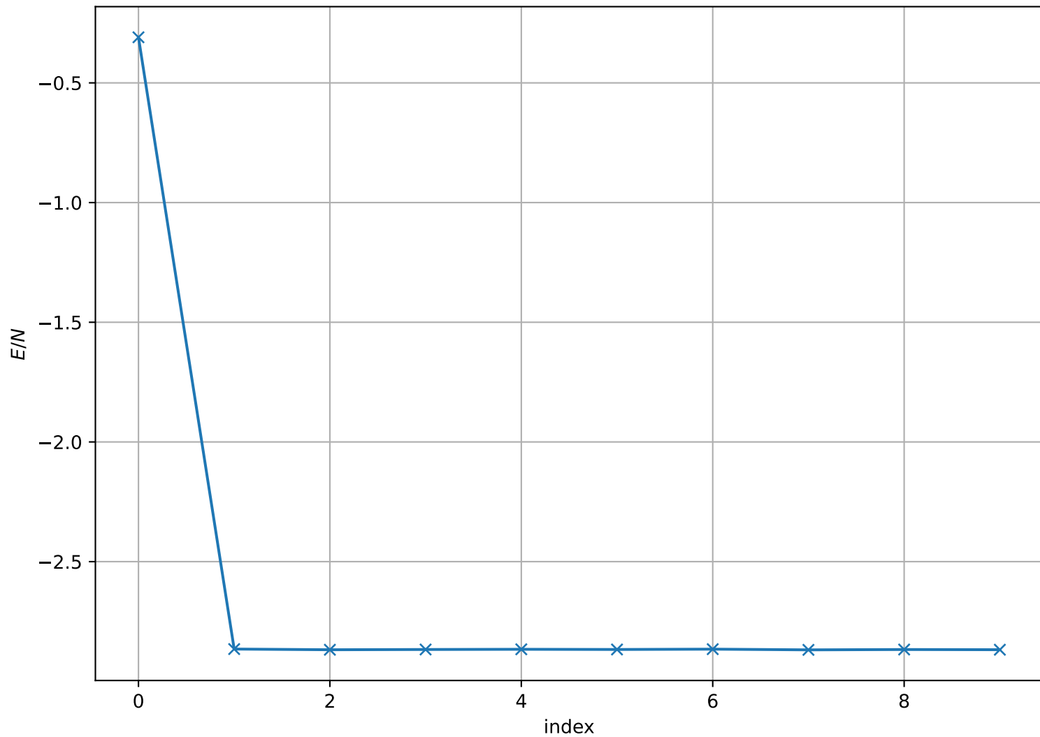
Energy per Site at T = 2.000e - 01 , L = 128
