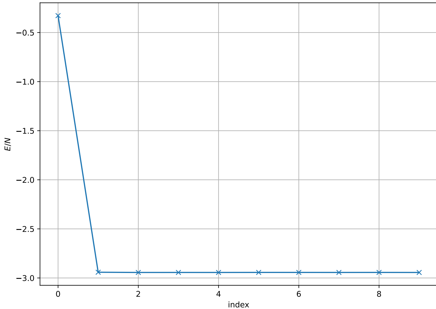
Energy per Site at T = 5.000e - 02 , L = 128
