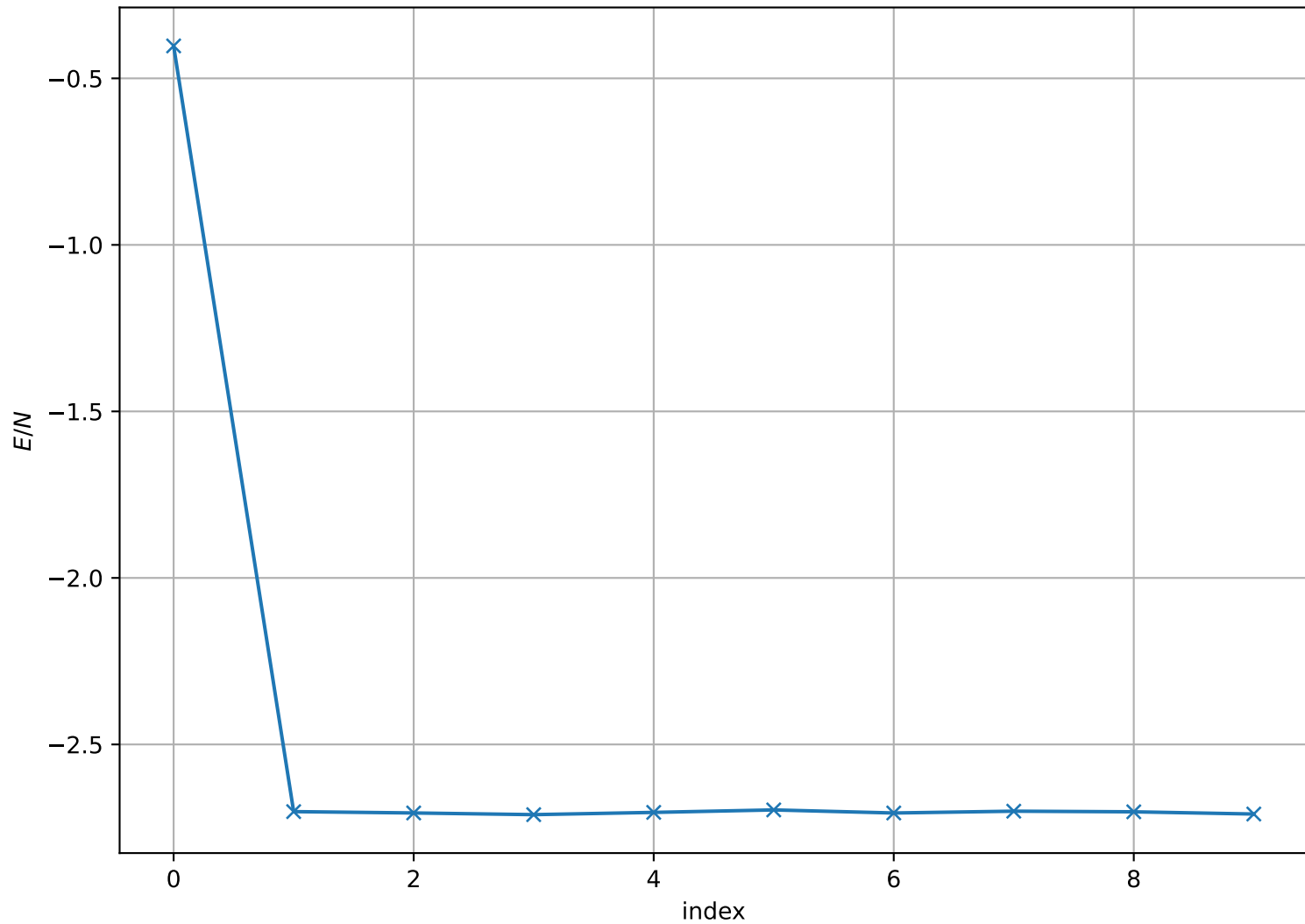
Energy per Site at T = 1.000e - 01 , L = 16
