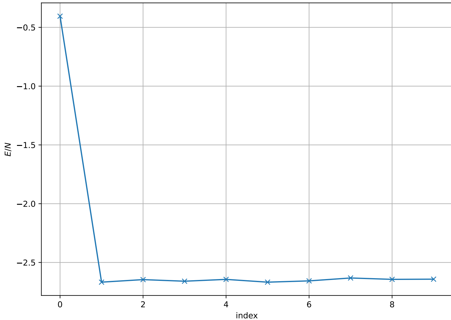
Energy per Site at T = 2.000e - 01 , L = 16
