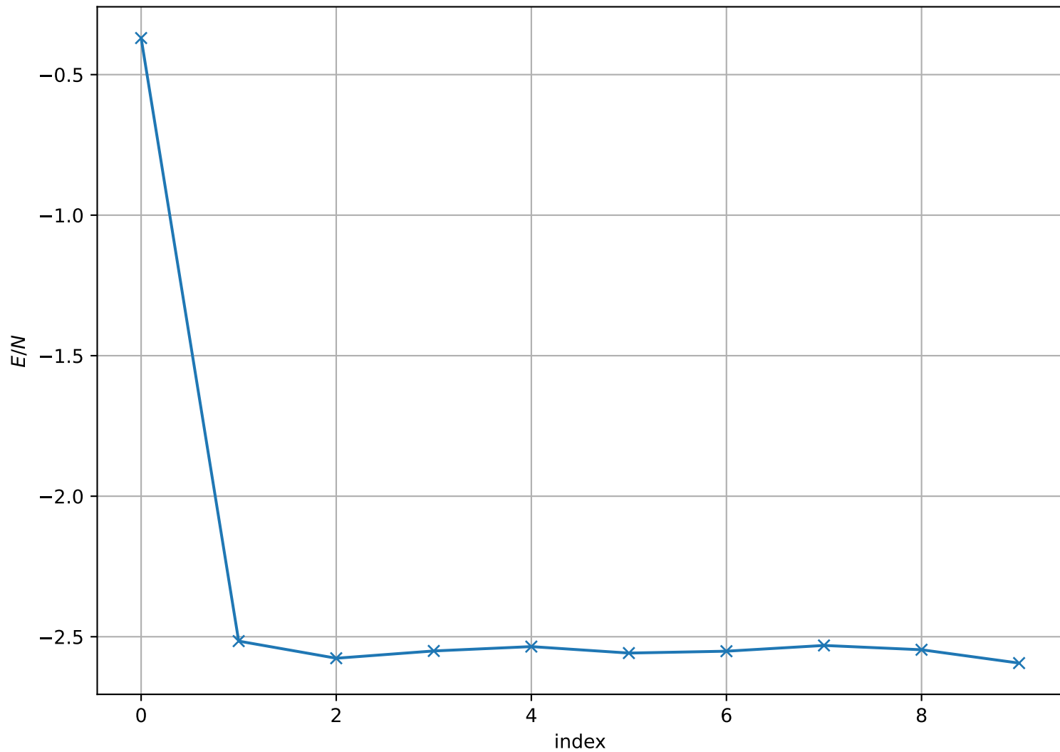
Energy per Site at T = 4.000e - 01 , L = 16
