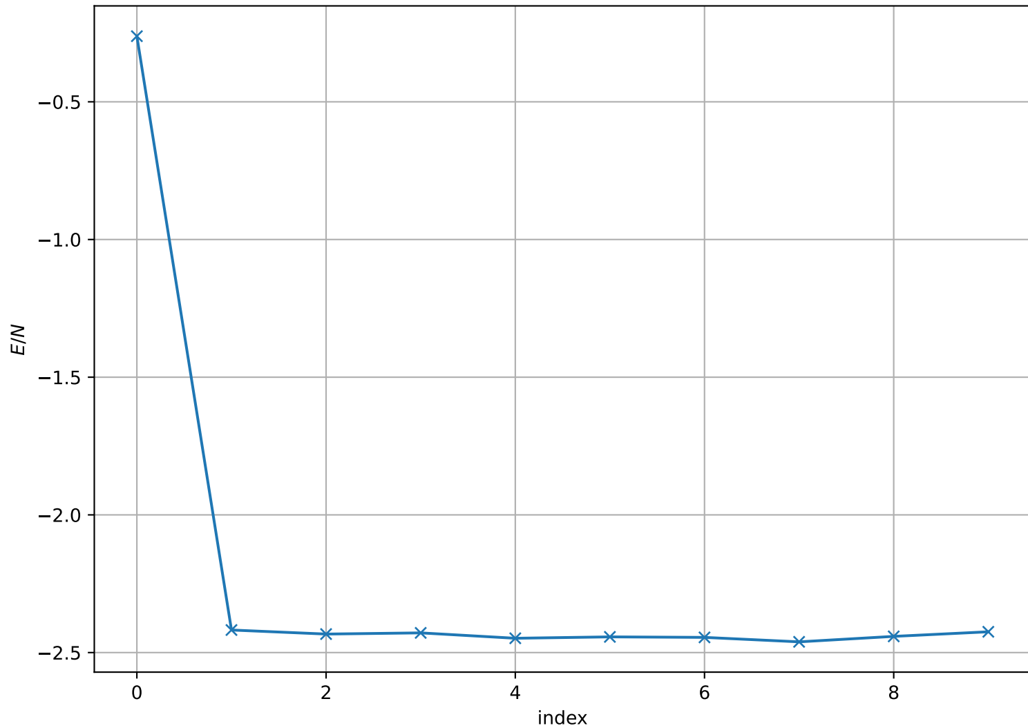
Energy per Site at T = 6.000e - 01 , L = 16
