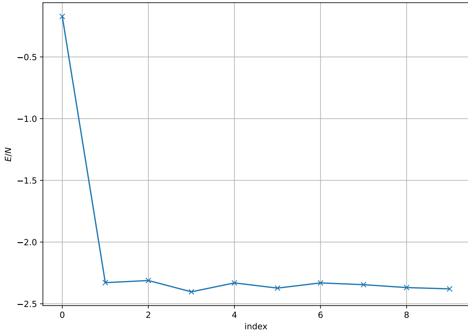
Energy per Site at T = 7.000e - 01 , L = 16
