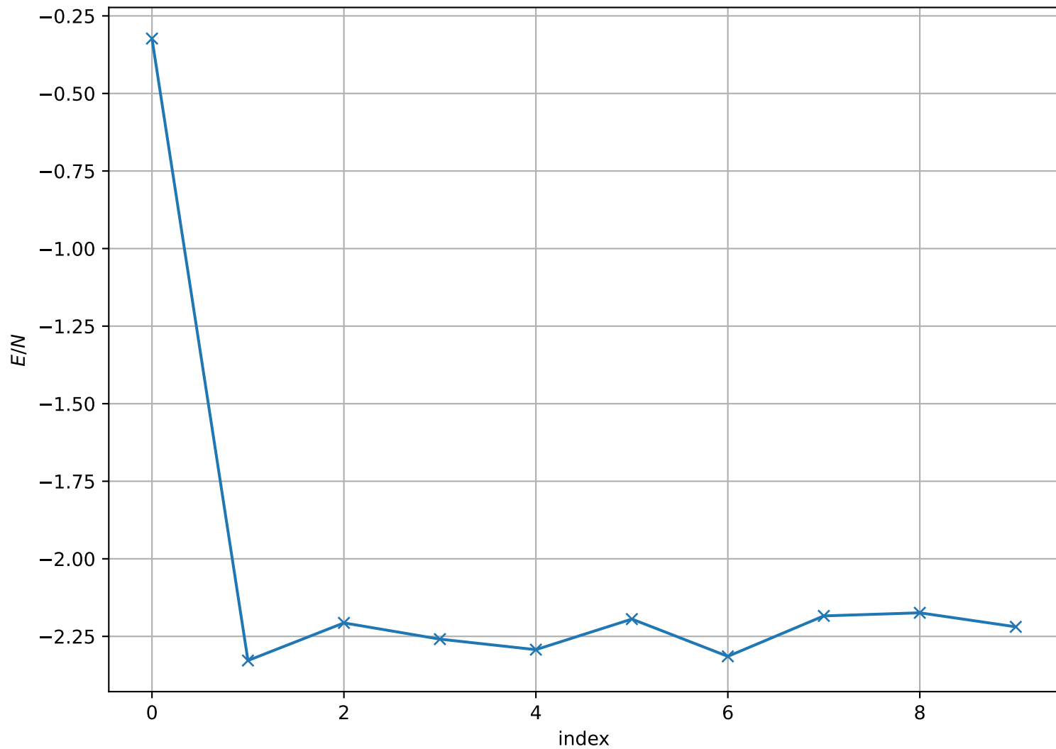
Energy per Site at T = 9.000e - 01 , L = 16
