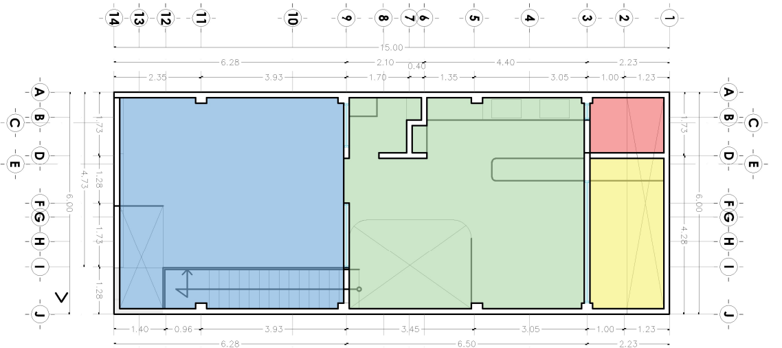
P I S O G E N E R A L P I S O C O C H E R A
