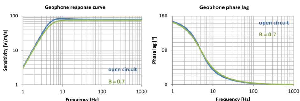
5Hz高灵敏度检波器幅度与相位响应曲线
