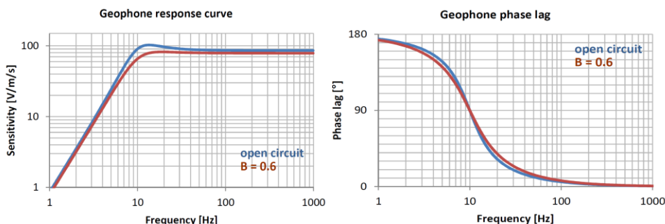
10Hz高灵敏度检波器幅度与相位响应曲线
