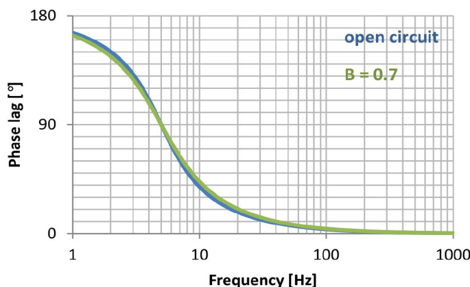
5Hz高灵敏度检波器幅度与相位响应曲线
