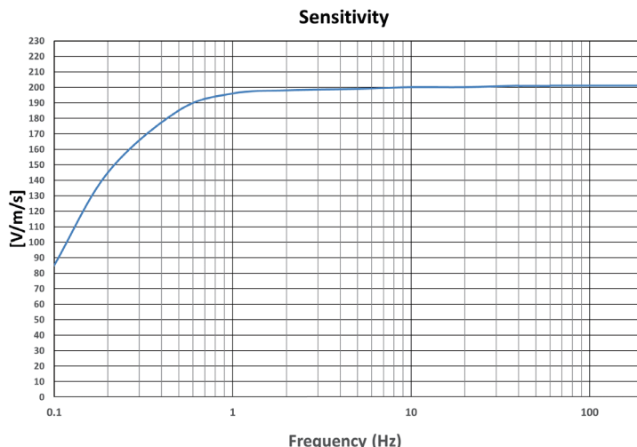
0.2Hz低频检波器幅频响应实测曲线
