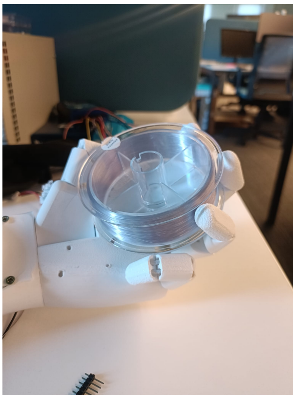
Figura 6.2: Mâna robotică prinzând un obiect cilindric.
