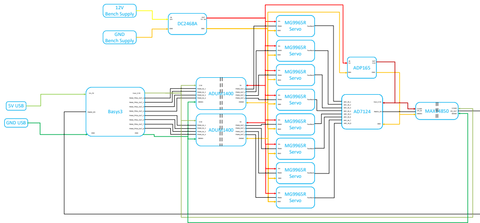
Figura 7.1: Schema conexiunilor dintre placa Basys3, izolatoare, convertor și servomotoare, cu alimentările aferente.
