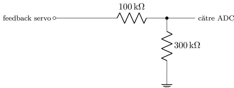
Figura 5.11: Schema unui divizor rezistiv de pe calea de feedback.
