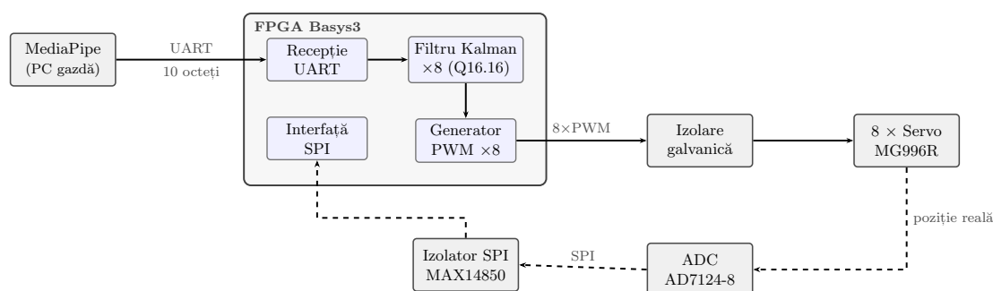
Figura 4.1: Structura logică a sistemului de control, cu fluxul principal de comandă (linie continuă) și bucla de monitorizare prin convertorul analog-digital (linie întreruptă).
